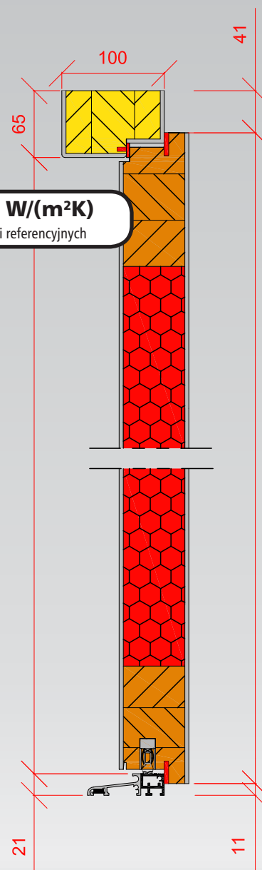
ALB-68 przekrój pionowy
